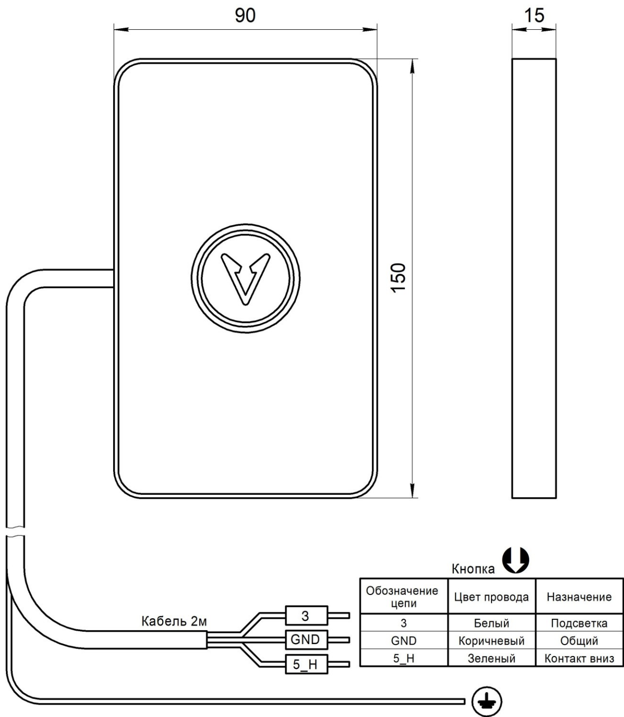
Рис.1 Внешний вид и габаритные размеры Вызывного поста ОНИКС НШЕК.468381.124
